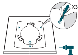
Otvor pre ethernetový kábel
